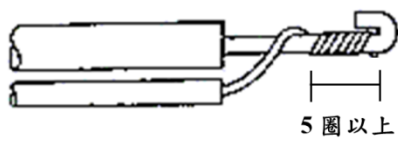
圖一五~十 不同線徑之實心線終端連接法
