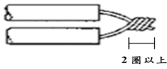
圖一五~九 實心線終端連接法
