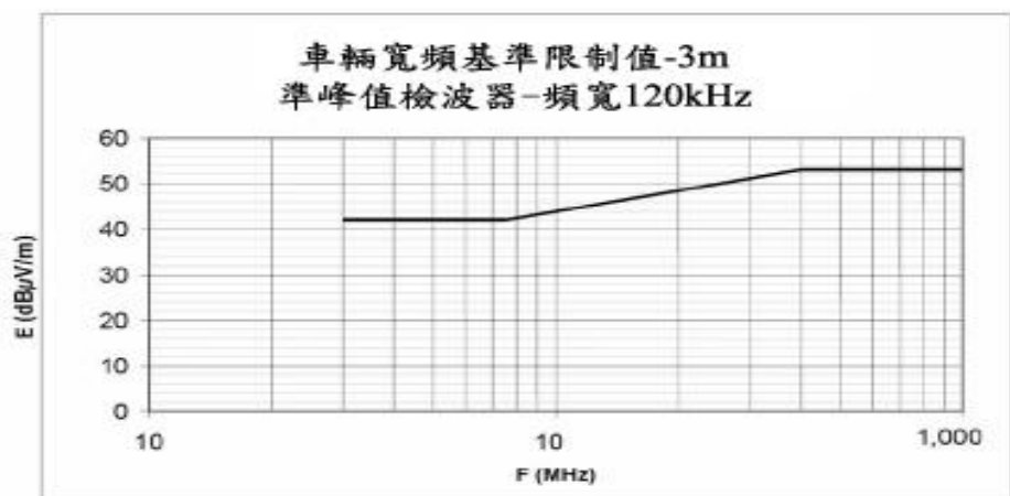
頻率-兆赫-對數 (參考本項4.2.2.2規定)
