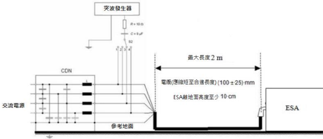
圖四十二：ESA 處於 REESS 充電模式連結電網之配置-交流（三相）電源線與接地線之間加以連結
