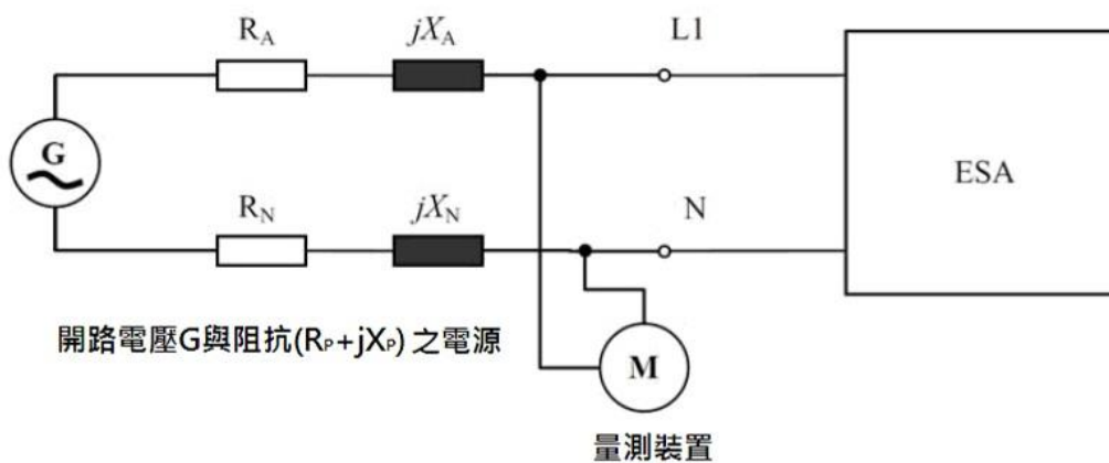
圖三十五之一：ESA 處於 REESS 充電模式連結電網之配置
