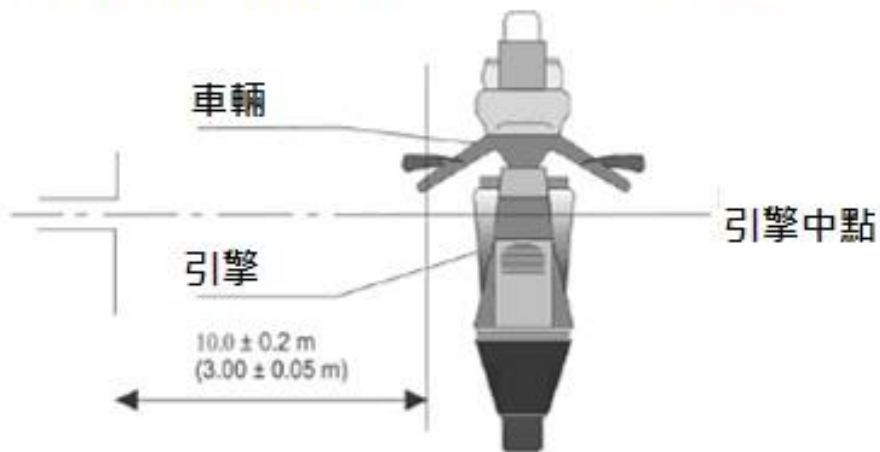
垂直極化量測示意圖
