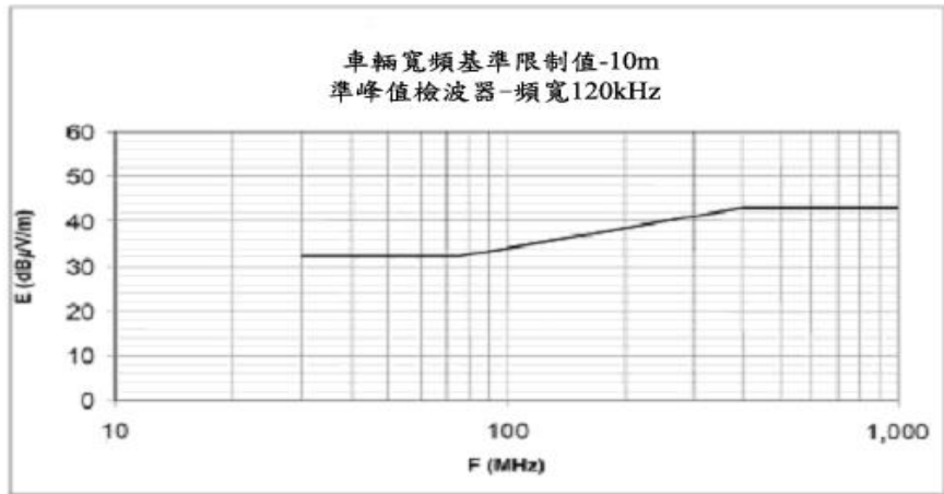
頻率-兆赫-對數 (參考本項4.2.2.1規定)
