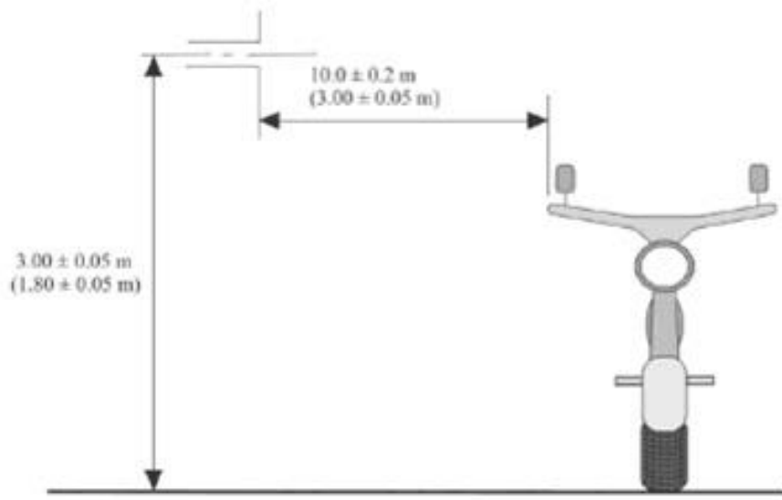
前視圖
