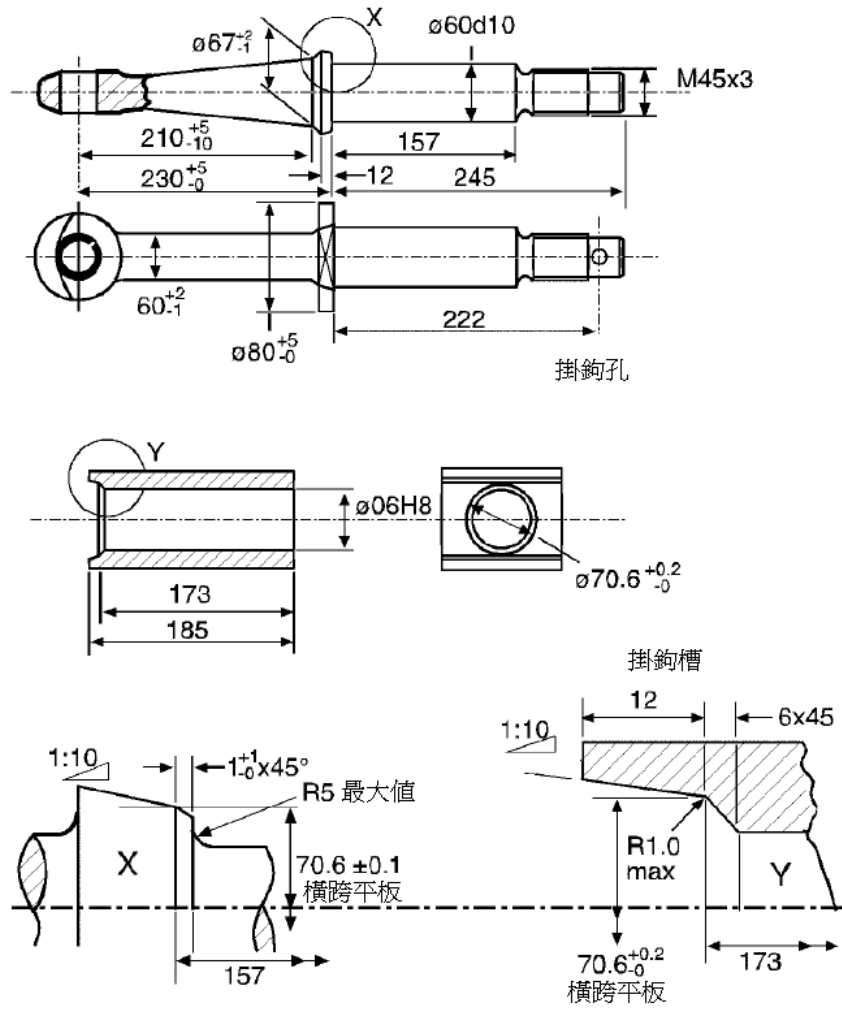
圖十二、類型 D50-B 掛鈎孔之尺寸(單位：公釐)
