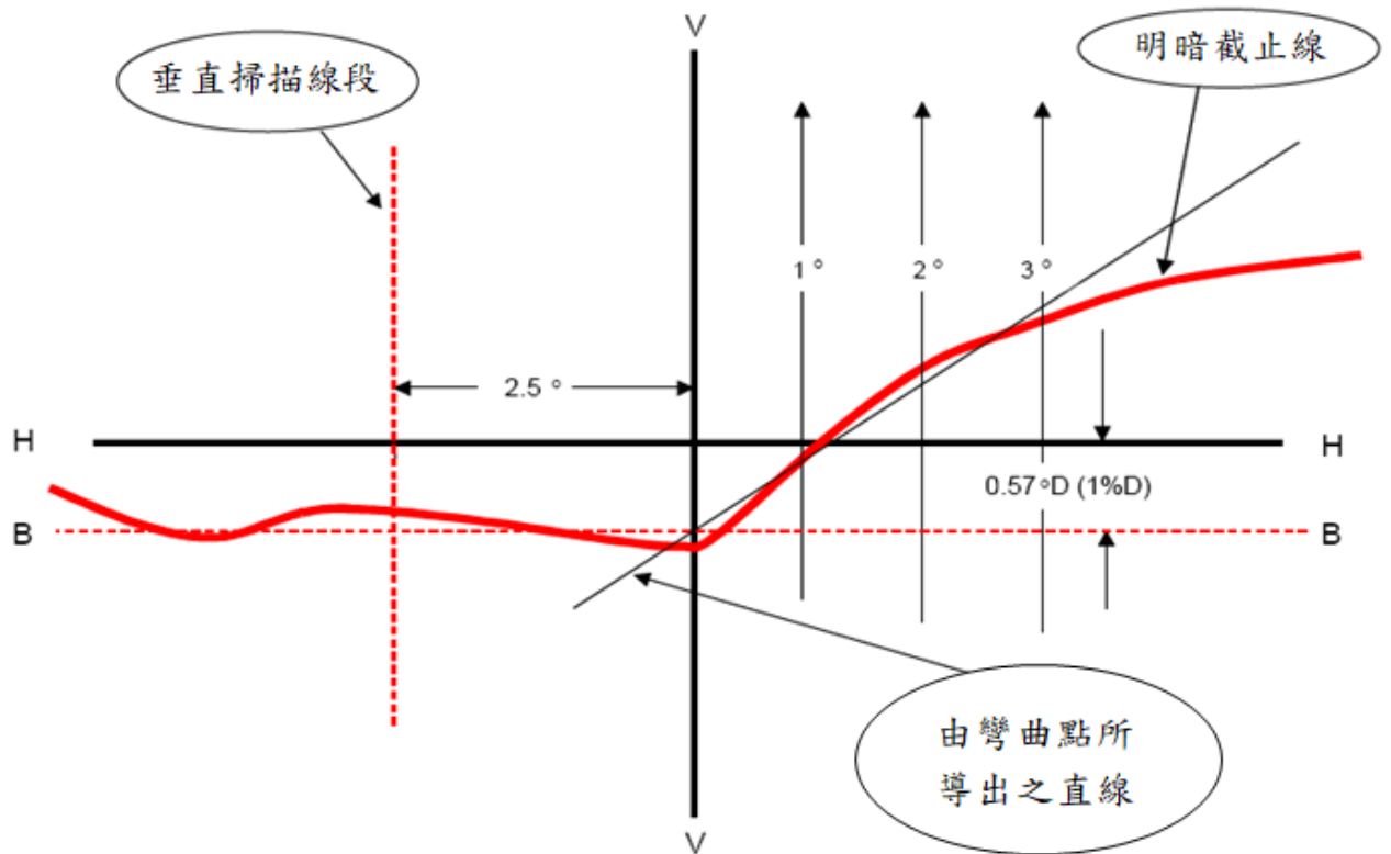
圖七：以儀器進行垂直及水平方向調整-三線段掃描法
