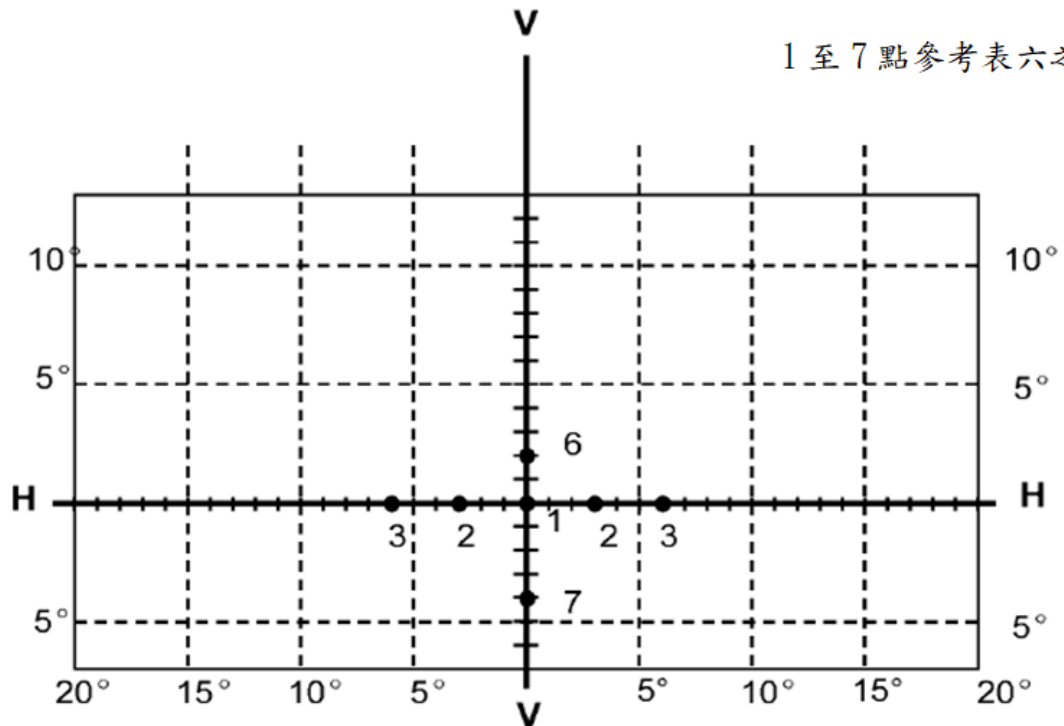
圖十：次要遠光燈
