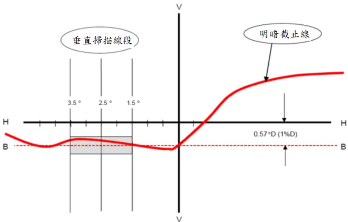
圖五：明暗截止線清晰度之量測
