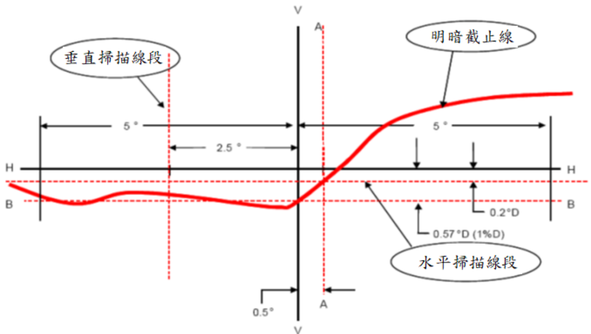
圖六：以儀器進行垂直及水平方向調整-水平線段掃描法
