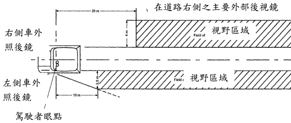
圖八：VII 類主要後方視鏡之地面視野區域
