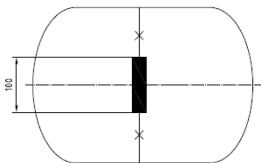
第八條圖十四 焊道照射長度：僅有一條周向接頭之鋼瓶
