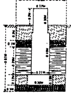
一等標石尺度 及埋設法
