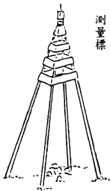
對角線四公尺 二三等點尋常方錐形木標
