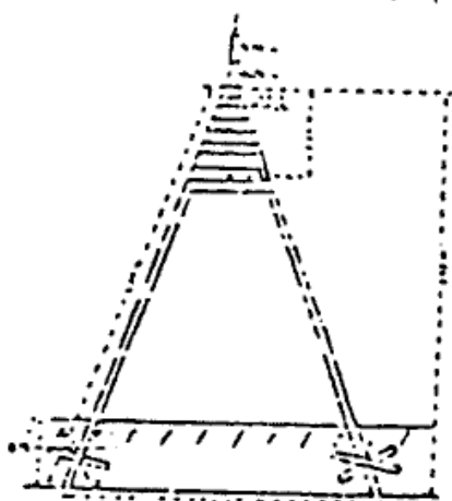
對角線四公尺 二三等點尋常方錐形木標
