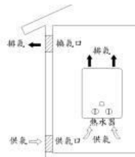
開放式熱水器（自然換氣方式）
