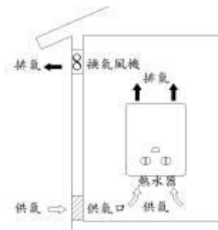
開放式熱水器（機械換氣方式）
