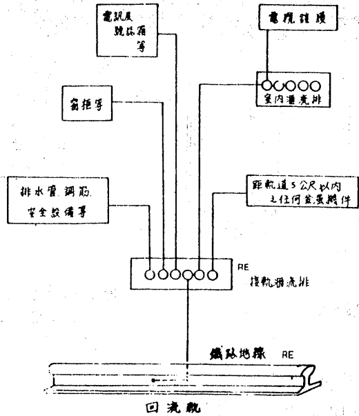
附圖二 臨近軌道各種金屬物體用接地線連結至回流軌之方塊示意圖
