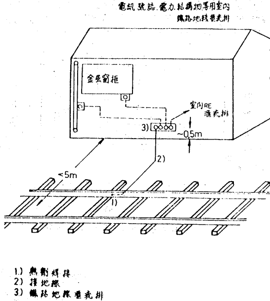
附圖三 臨近軌道建築物內各種金屬物件藉滲漏排及共同接地線連結至回流軌之情形
